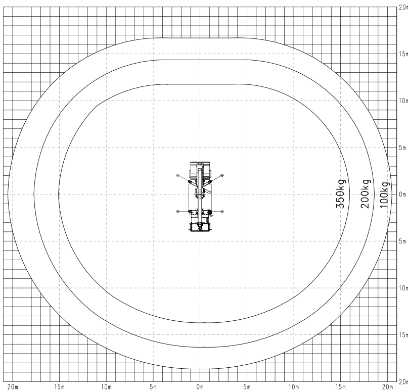
Abstützbreite variabel
