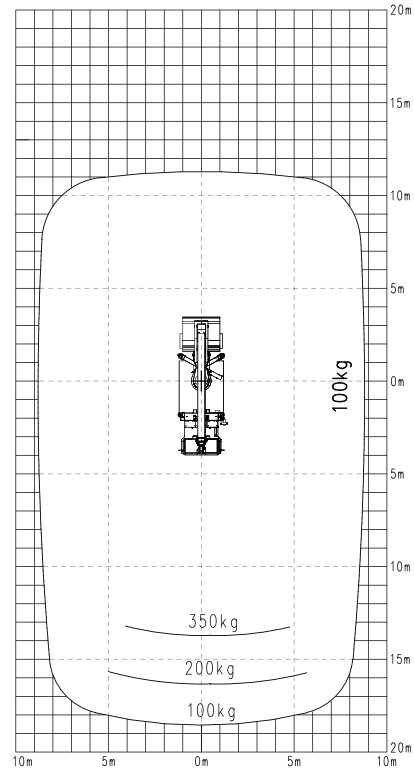
Abstützbreite schmal
