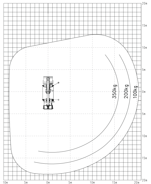
Abstützbreite einseitig
