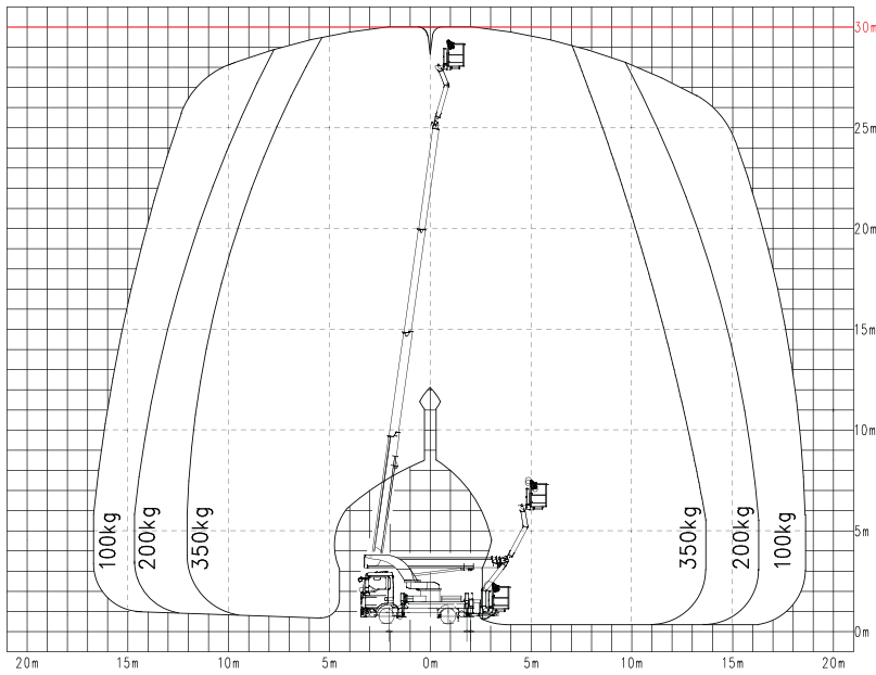
Abstützbreite variabel
